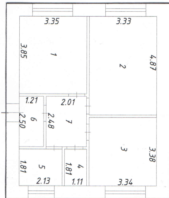
План здания
