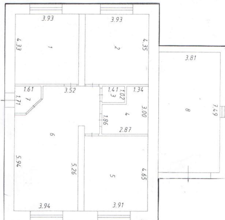
План здания
