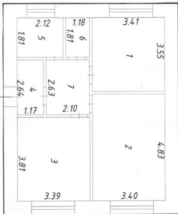
План здания
